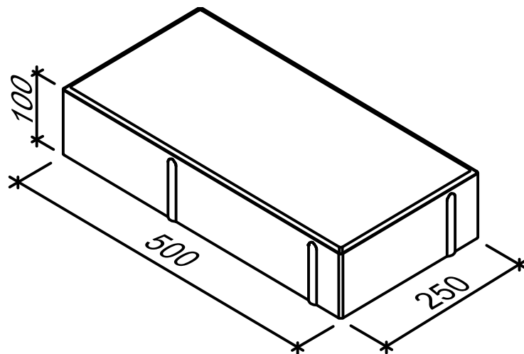
Obr. č. 3 Přídlažba 8 - rozměry
