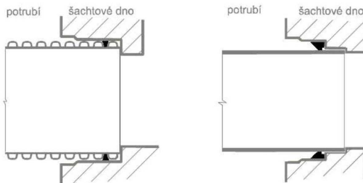
obr. Správné uložení potrubí k dorazu přejíždky v šachtovém dně
