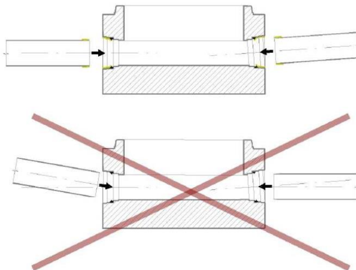
obr. Zasunutí potrubí do šachtové přechodky správně/špatně
