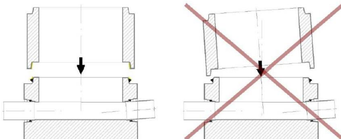
obr. Sestavení šachty správně/špatně
