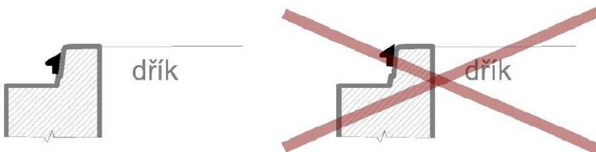
obr. Nasazení šachtového těsnění správně/špatně
