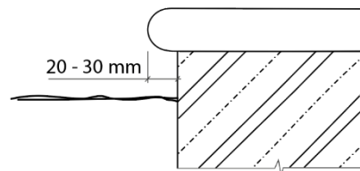
Obr. č. 13 Detail přesahu bazénových lemů
