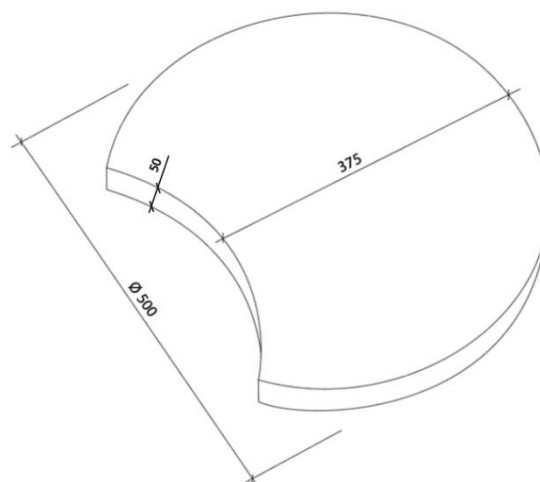
Obr. č.3 Nášlap s výsečí 50 - průběžná;
