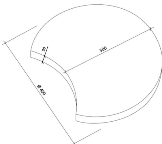
Obr. č. 2 Nášlap s výsečí 40 - průběžná
