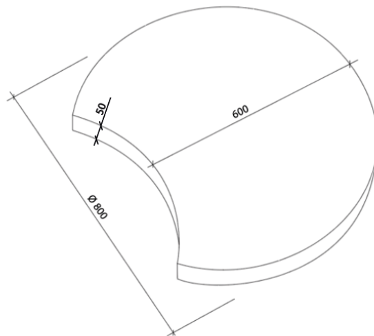
Obr. č. 5 Nášlap s výsečí 80 průběžná
