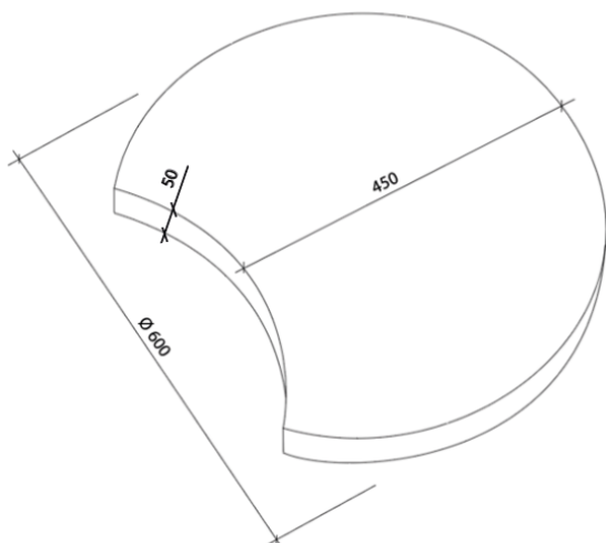
Obr. č. 4 Nášlap s výsečí 60 - průběžná
