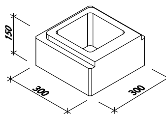
Obr. č. 6 Verso koncový poloviční
