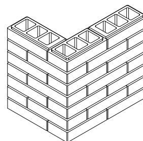
VERSO SKLADBA ROH
